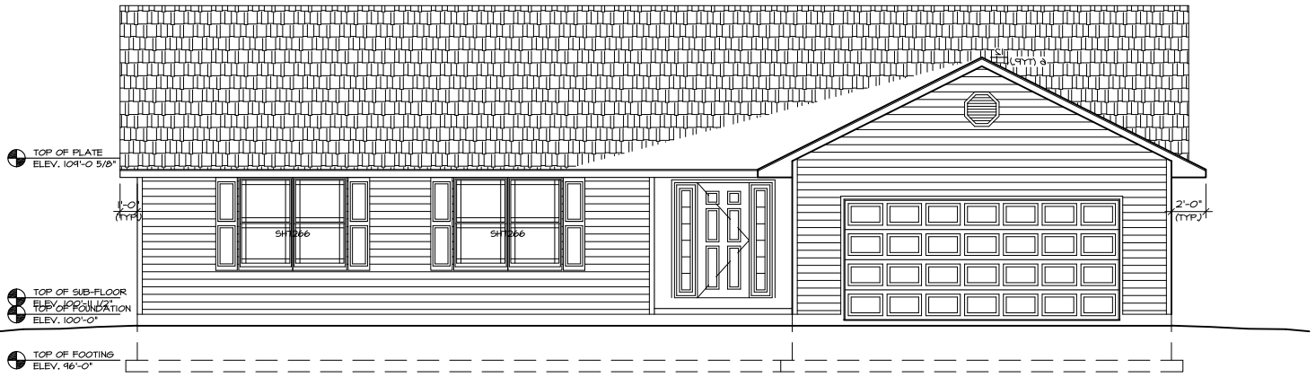
I FRONT ELEVATION A-1 SCALE: 1/4"=1'-0"
